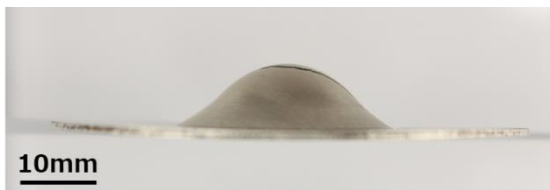
図3 ZA系新合金圧延材の室温エリクセン試験結果
