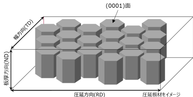
図1 一般的なマグネシウム合金圧延材の結晶組織の配向
